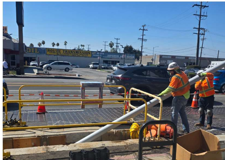
Trabajo de instalación de conductos en Van Nuys Bl y Keswick St
