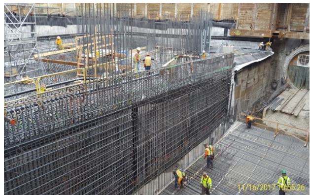
Rebar installation and preparation for wall pour
