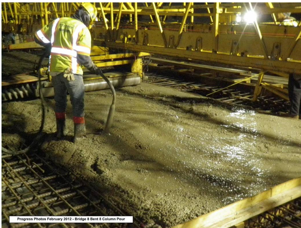
Bridge 8 Bent 8 column pour.
