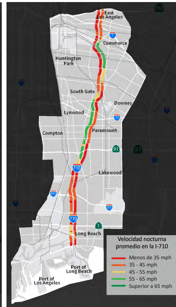
Figura 3-66. Velocidad Nocturna en la Autopista I-710
