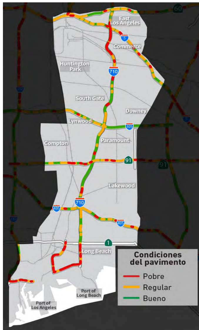
Figura 3-70. Condiciones del Pavimento de la Autopista
